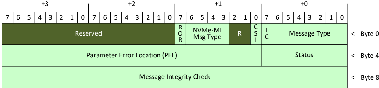
Figure 30: Invalid Parameter Error Response
